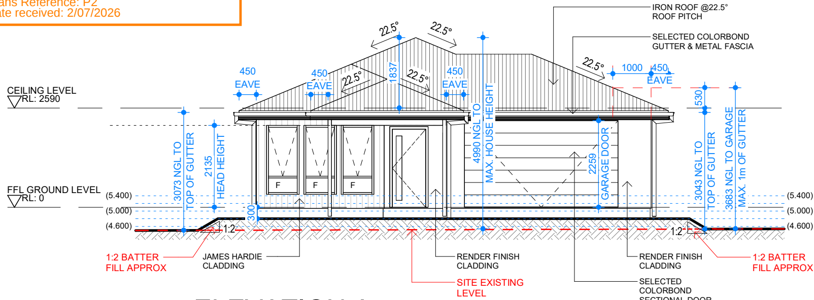
ELEVATION A
