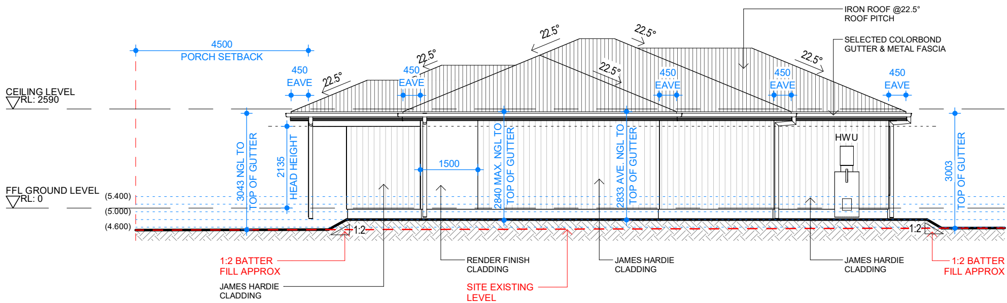
ELEVATION D 1 : 100
