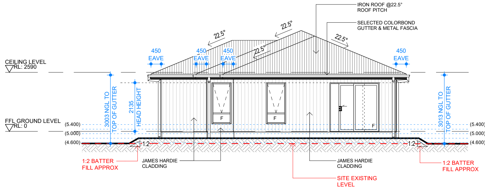
ELEVATION C 1 : 100
