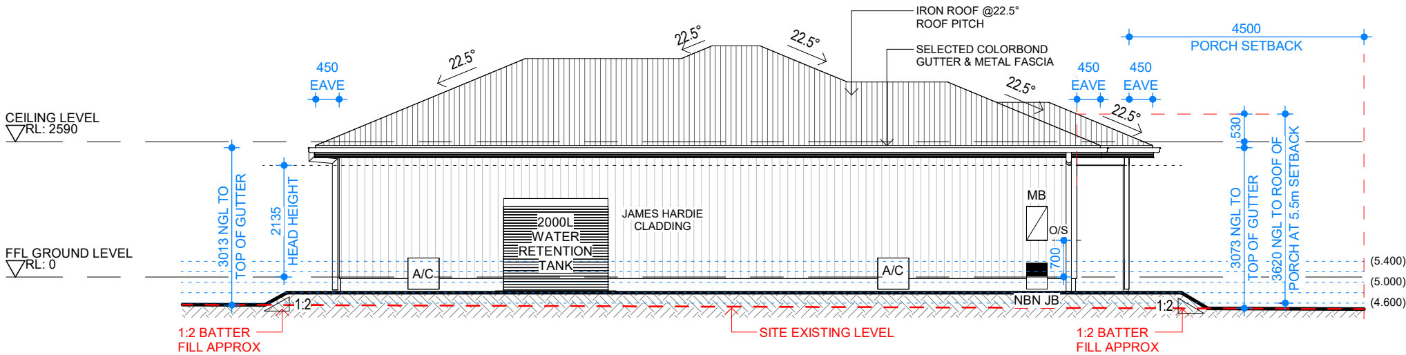
ELEVATION B
